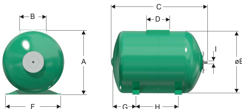
Dimensiones Generales
