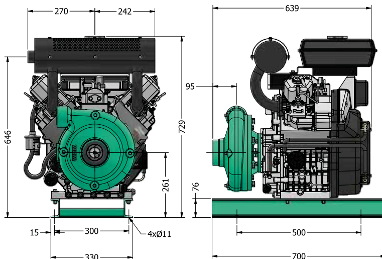
DIMENSIONES EN MILIMETROS
