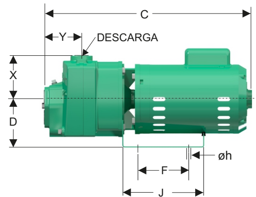
DIMENSIONES EN MILIMETROS
