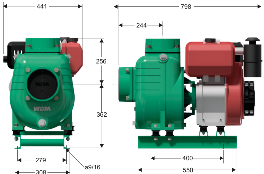
Dimensiones en milímetros
